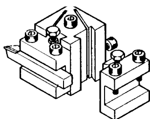
Tourelle livrée avec 2 porte-outils.
