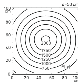
Exemple : éclairage 1 x 36 W avec grille parabolique
