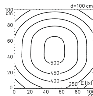
Exemple : éclairage 2 x 36 W avec grille parabolique (112 449 011 - 000 813 32)
