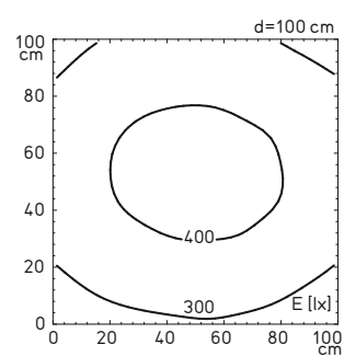
Exemple : éclairage 30 W
