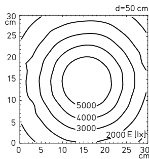
Éclairage avec optique 40°
