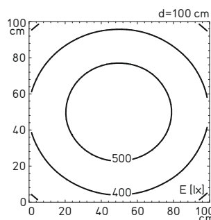
Exemple : éclairage 24 W sans optique (95°)
