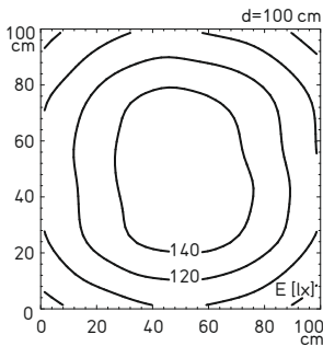
Éclairage AWDCE avec réflecteur
