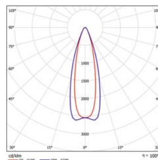
Diffusion très étroite pour hauteurs de hall d'env. 10–18 m, optique xN
