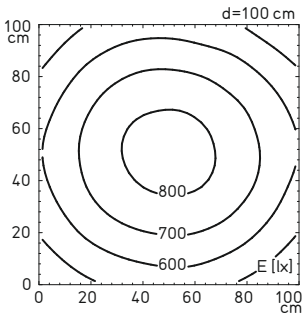
Exemple : éclairement 21,5 W
