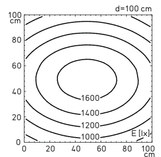
Exemple : éclairage 1 x 54 W T5
