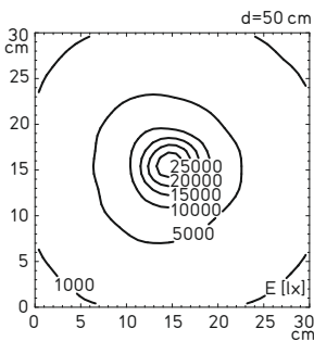
Éclairage avec optique 10°
