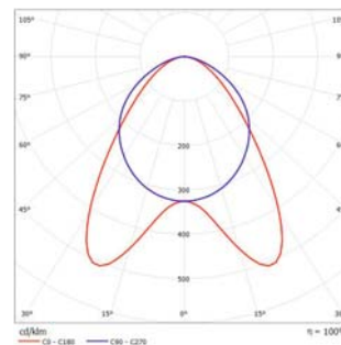
Doublement asymétrique pour les entrepôts, optique D
