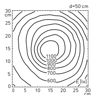
Éclairage avec optique 25°
