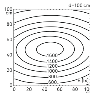
Exemple : éclairage de la MLAL 57 S avec optique 40°
