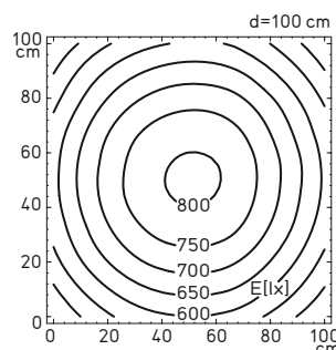
Exemple : éclairage 2 x 39 W sans grille parabolique
