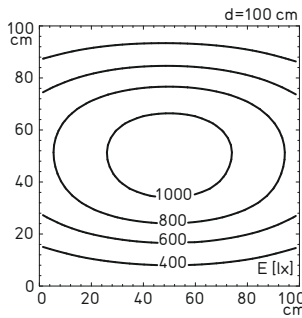
Exemple : éclairage 24 W avec optique 30°
