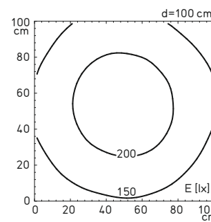
Exemple : éclairage 10 W avec tube de luminaire blanc opale
