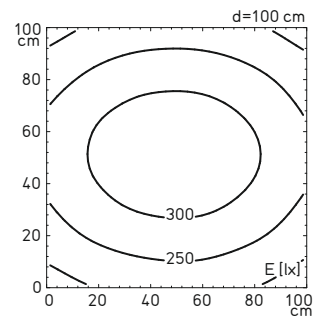
Exemple : éclairage 28 W avec diffuseur transparent
