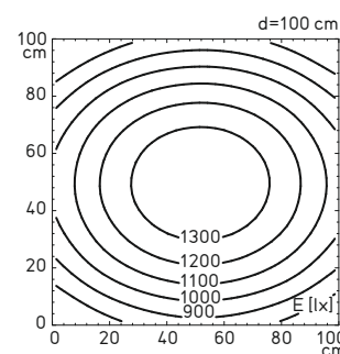
Exemple : éclairage de la MQAL 84 S
