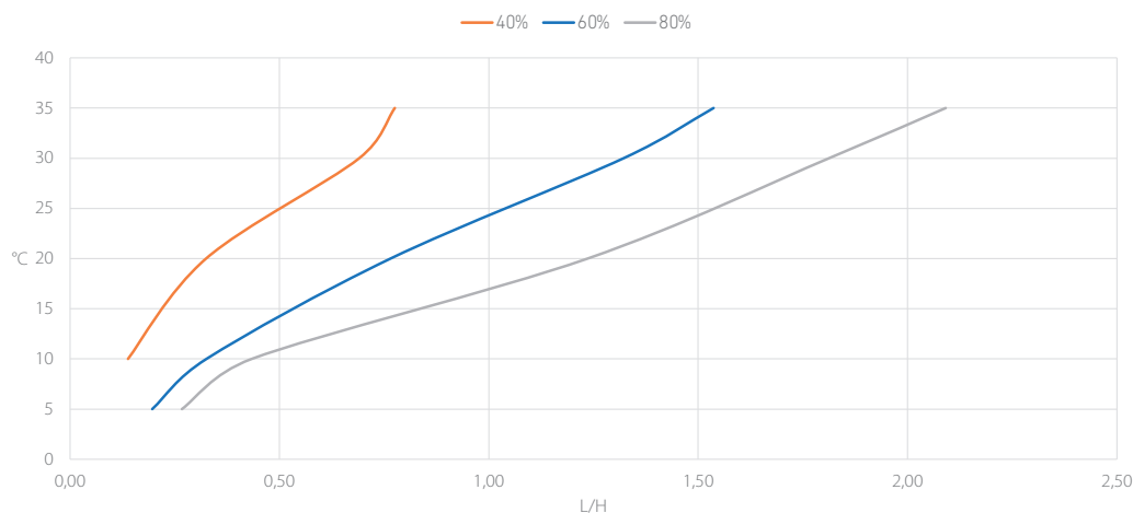
CDT40 MKIII : COURBES DES CAPACITÉS
